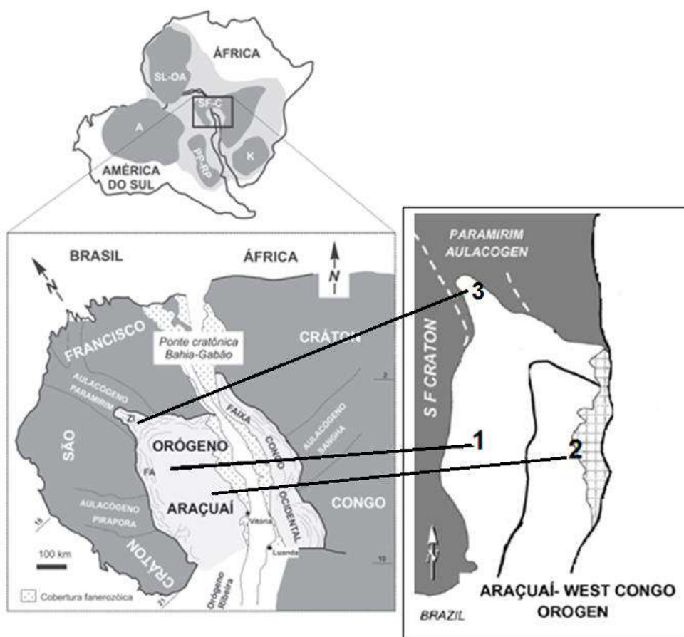
Figura 3. O Orógeno Araçuaí na região central do Paleocôntinente; Domínios tectônicos do Orógeno Araçuaí, (1) domínio externo, (2) domínio interno, (3) Zona de Inflexão. Fonte: Modificado de Alkmim et al. (2006) e Pedrosa-Soares et al. (2007).
