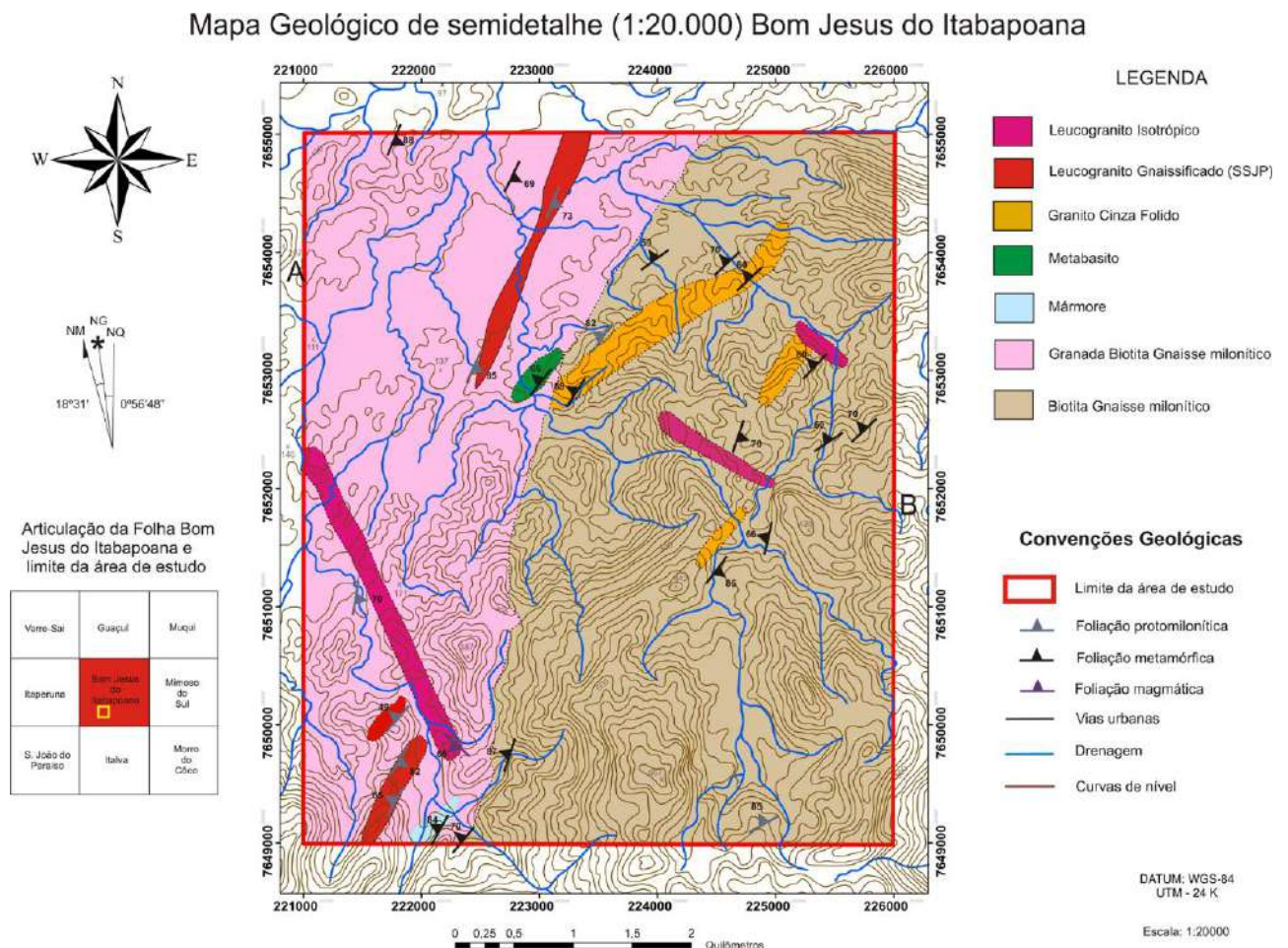
Figura 1: Mapa Geológico de Semidetalhe (1:20.000) nas Proximidades de Bom Jesus do Itabapoana – RJ.
