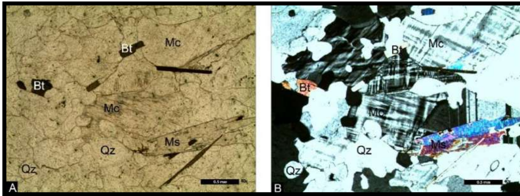
Figura 3: Visão petrográfica do microclina gnaisse com a distribuição dos minerais essenciais: microclina (Mc), quartzo (Qz), plagioclásio (Pl), muscovita (Ms) e biotita (Bt). A- LPP; B-LPX.
