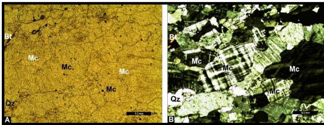
Figura 4: Contatos do tipo interlobados entre os grãos do microclima gnaisse. A- LPP; B-LPX.
