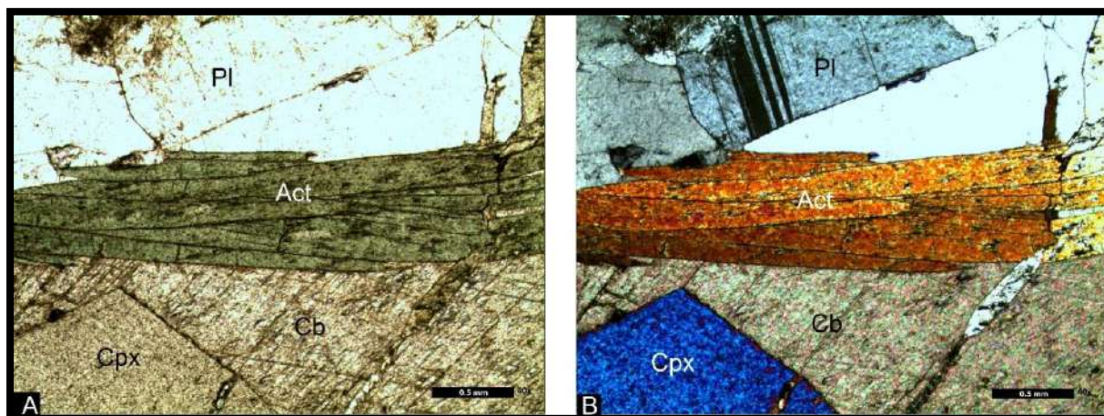
Figura 10. Clinopiroxênio-plagioclásio granofels: plagioclásio (Pl), clinopiroxênio (Cpx), actinolita (Act) e carbonato (Cb). A- LPP; B-LPX.
