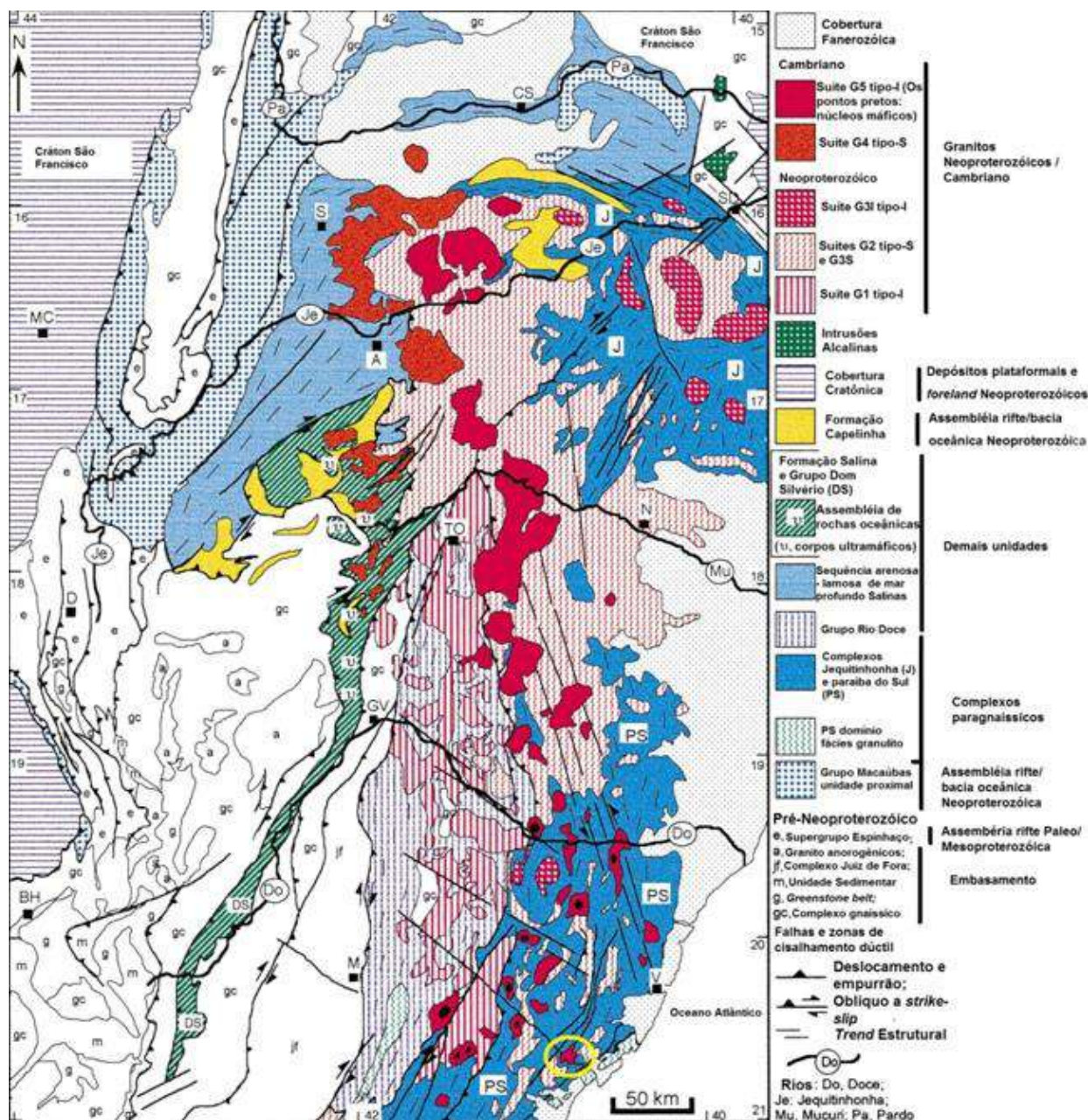
Figura 4. Mapa geológico mostrando os componentes litotectônicos no Orógeno Araucaí, uma visão geral de um orógeno confinado formado durante a montagem Gondwana, com a área de estudo marcada em amarelo. Fonte: Modificado de Pedrosa-Soares et al. (2001).
